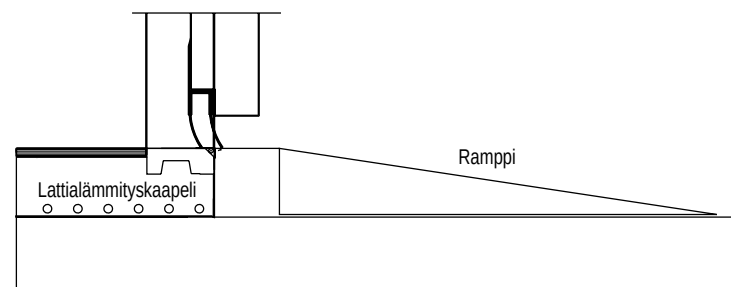
Rakennuksen lattian päällinen lattiaelementti ja ramppi
