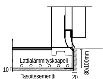
Upotettu lattiaelementti
