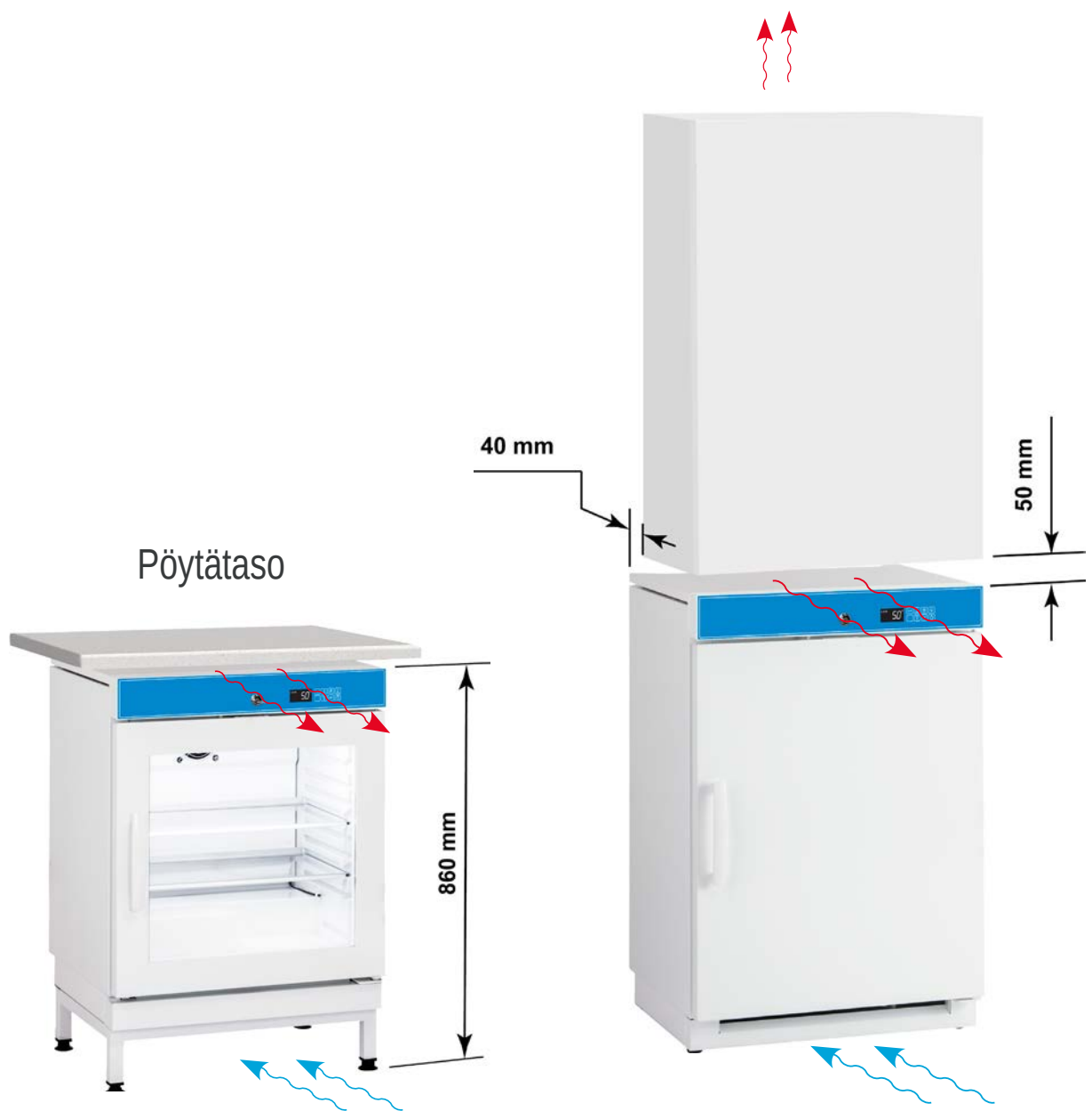
Asennus pöytätason alle
