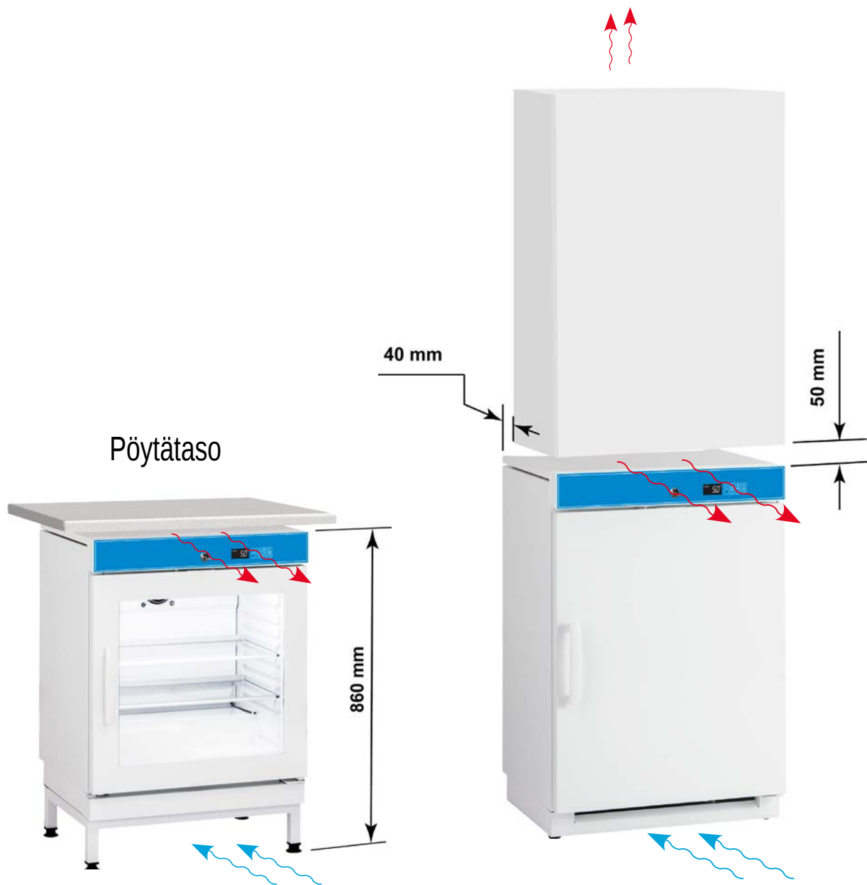
Asennus pöytätason alle
