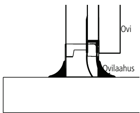
Ilman lattiaelementtiä
