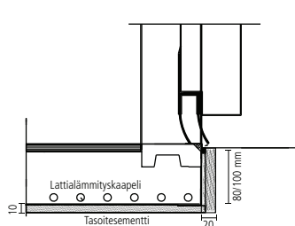
Upotettu lattiaelementti
